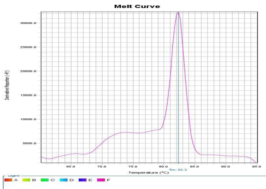
شکل ۲- نمونه نمودار منحنی دمای ذوب ژن IDE
